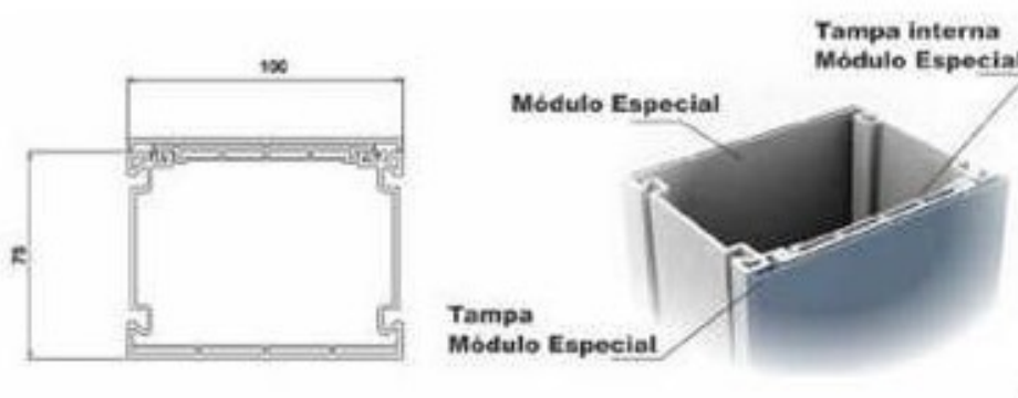
FIGURA 6 – Módulo especial usado para passagem de tubulações hidráulicas
