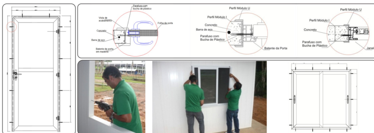
FIGURA 8 – Detalhamento de fixação das portas e das janelas
