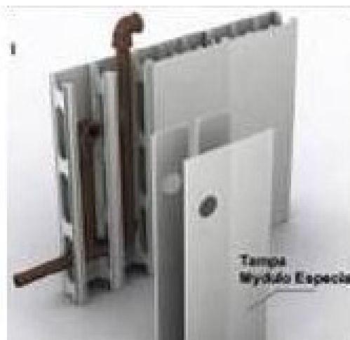
FIGURA 7 – Vista de uma parede com tubulação inserida nos módulos especiais
