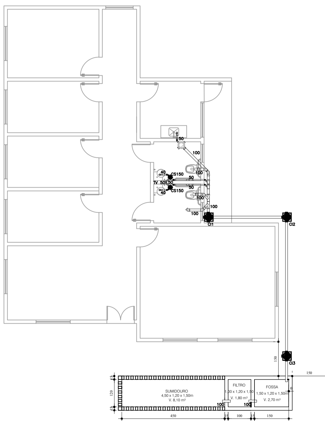
PLANTA BAIXA HIDROSSANITÁRIO ESC:1/100
