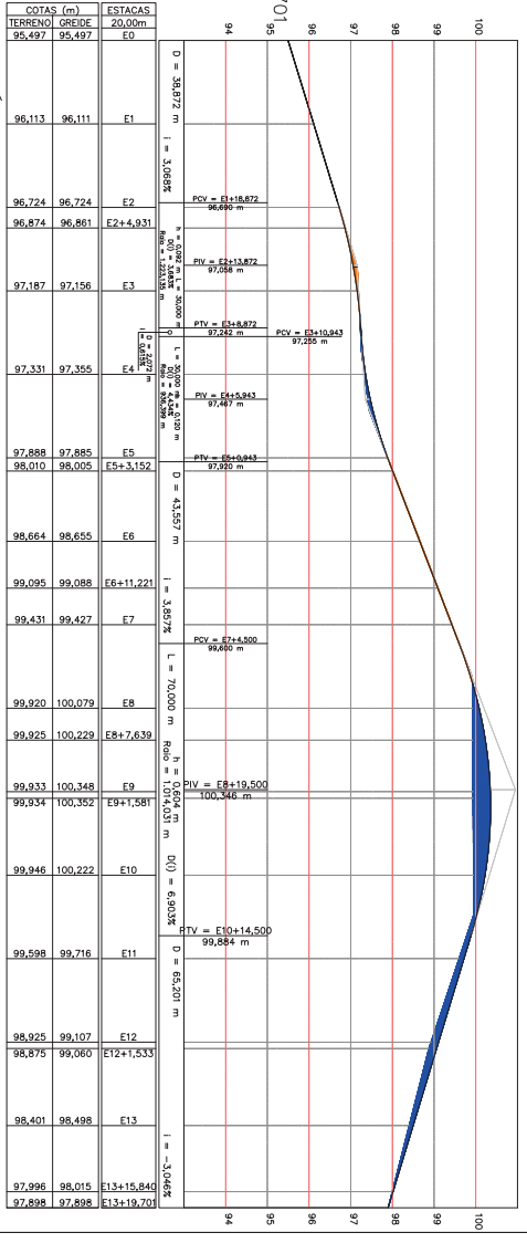
GEOMÉTRICO Perfil Longitudinal Escala H=1:50 V=1:50
