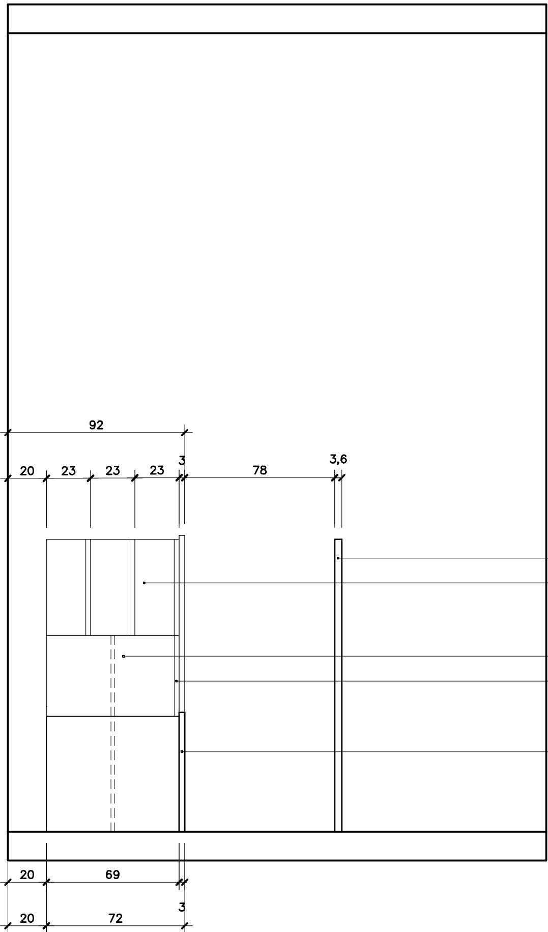
VISTA B - Esc: 1/20
