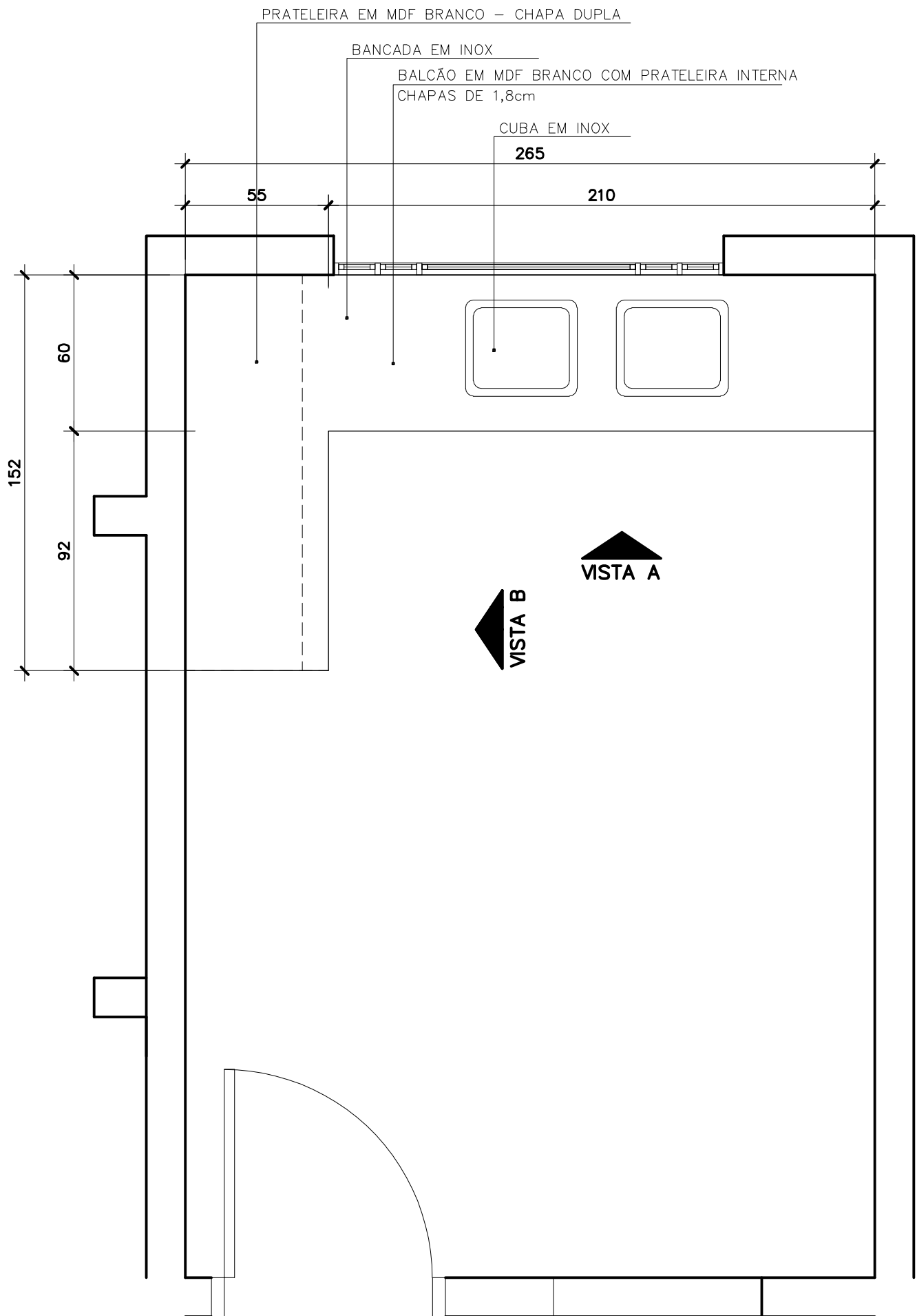
PLANTA BAIXA COZINHA SÃO FELIPE – Esc: 1/20
